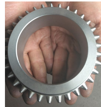
歯面取り(チャンファ)加工後
